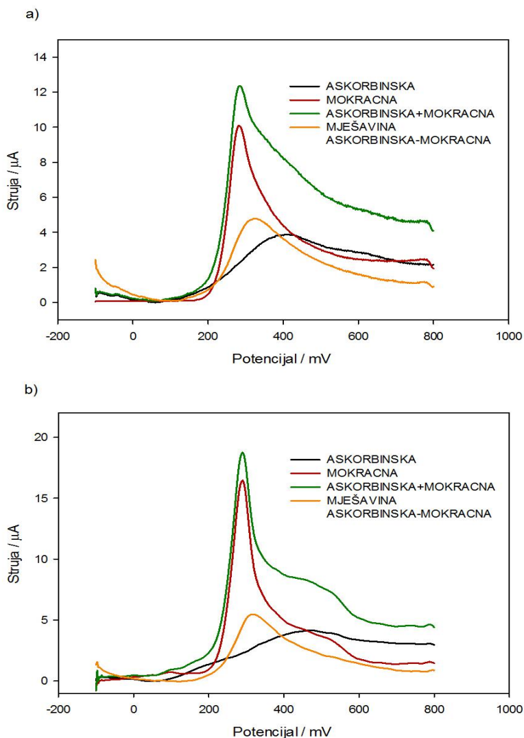
Slika 4.7. Odziv mješavine askorbinske i mokraćne kiseline u usporedbi sa odzivima pojedinačnih kiselina te zbrojem njihovih signala pod a) sobnim osvijetljenjem i b) UV lampom
