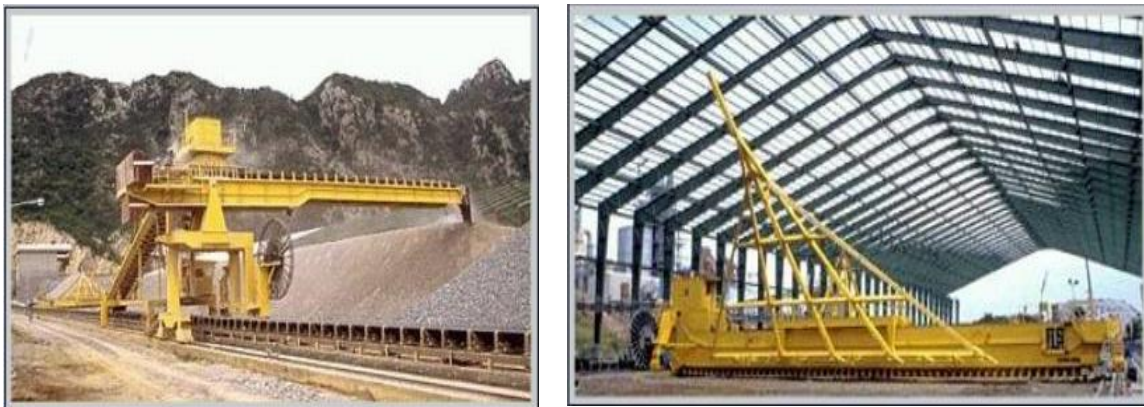
Slika 2. Predhomogenizacija sirovine
