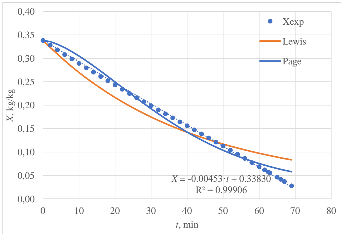
Slika 30. Aproksimacija eksperimentalnih podataka Lewisovim i Pageovim modelom ( T=45\text{ °C} )
