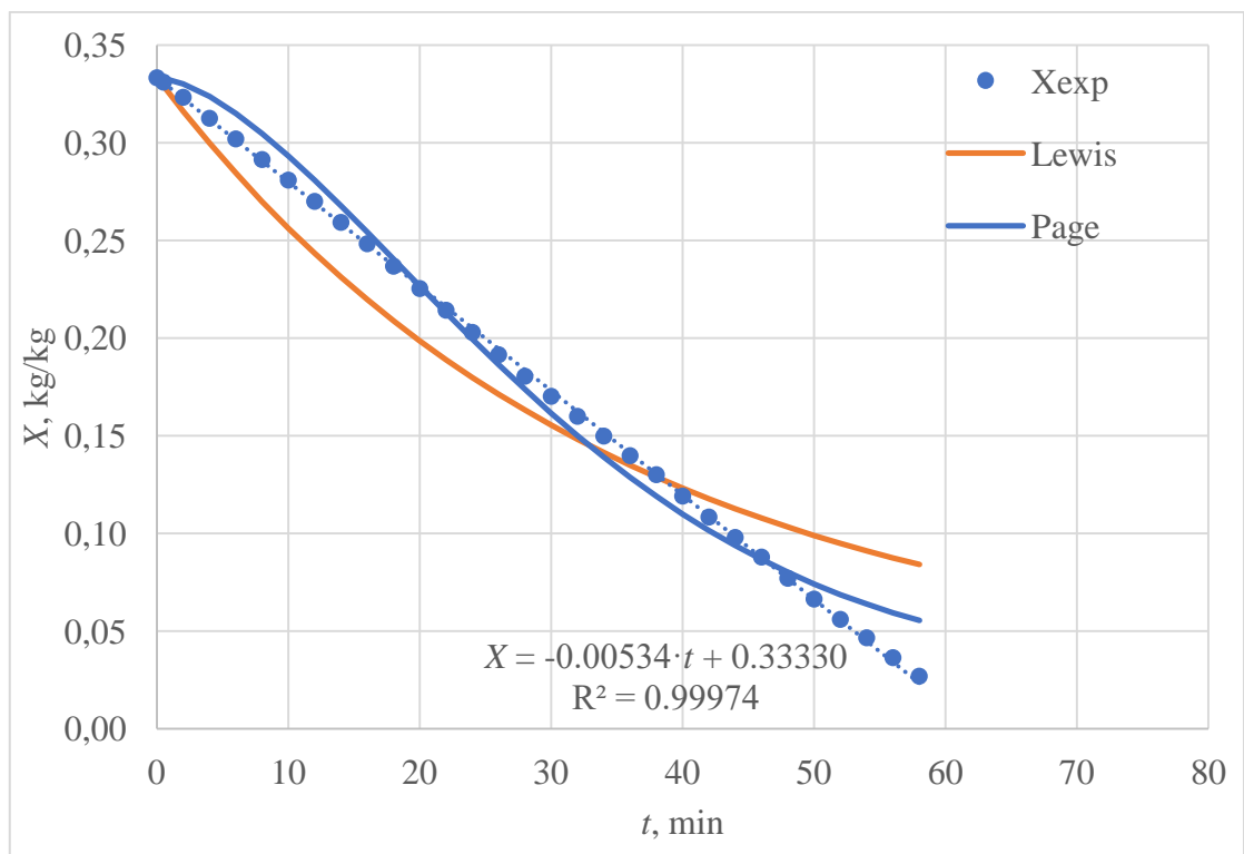
Slika 31. Aproksimacija eksperimentalnih podataka Lewisovim i Pageovim modelom ( T=60\text{ °C} )
