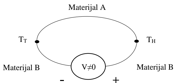
Slika 2. Shematski prikaz Seebeckovog efekta
