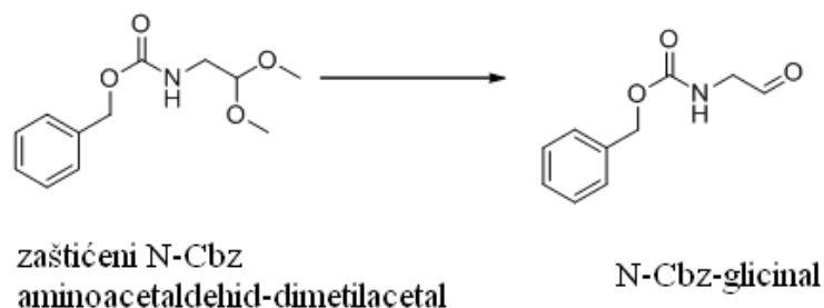
Slika 3.7. Reakcija odštićivanja N-Cbz-glicinala
