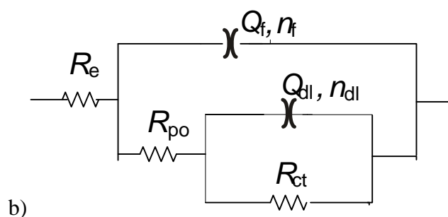
Slika 19. Električni ekvivalentni krugovi korišteni za modeliranje eksperimentalnih podataka
