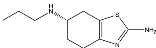
Slika 13. Struktura pramipeksola
