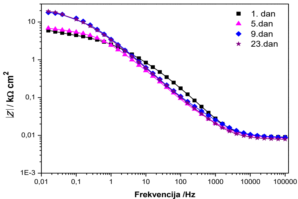
Slika 15. Bodeov prikaz impedancijskih krivulja za uzorak kod kojeg se adsorpcija odvijala u otopini ODPA koncentracije c(\text{ODPA}) = 10^{-4} \text{ M} u ovisnosti o vremenu izlaganja 3%-tnoj otopini NaCl-a.
