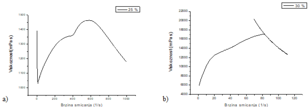
Slika 19. a) Grafički prikaz ponašanja viskoznosti s povećanjem brzine smicanja za 25 %-tni nanofluid b) Grafički prikaz ponašanja viskoznosti s povećanjem brzine smicanja za 30 %-tni nanofluid
