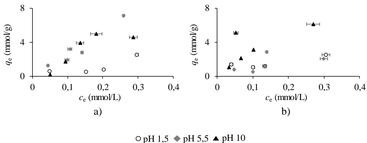
Slika 44 Adsorpcijska ravnoteža za adsorpciju cijanidin-3-glukozida (a) i cijanidin-3-galaktozida (b) na \beta -glukanu na pH 1,5, 5,5 i 10,0
