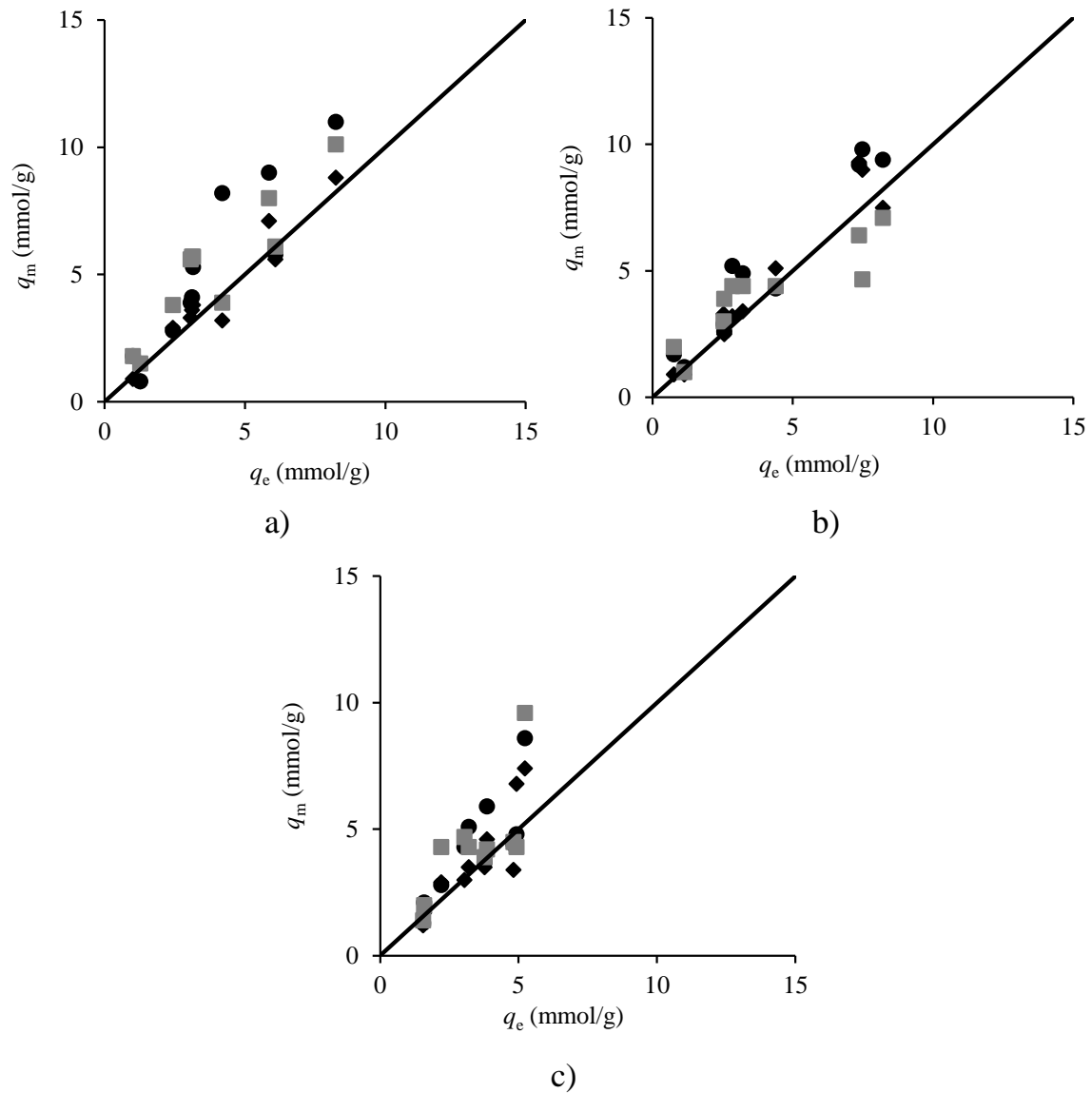
Slika 20 Odnos adsorpcijskih parametara q_m iz Langmuirrove (●), Dubinjin-Raduškjevičeve (◆) i Hillove izoterme (■) naspram eksperimentalno određenih adsorpcijskih kapaciteta polifenola q_e . Prikazani rezultati odnose se za početne koncentracije od 150 mg/L, pH-vrijednost medija 5,5 te temperature: a) 25 °C, b) 37 °C i c) 45 °C.
