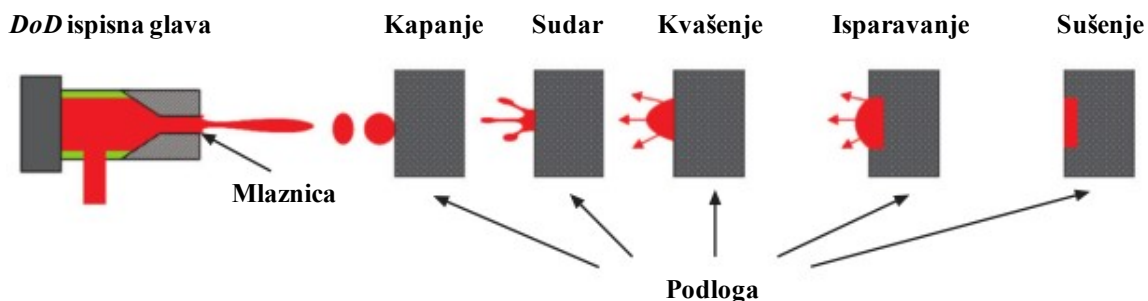
Slika 22. Shematski prikaz ispisivanja vodljive suspenzije DoD tintnom tehnologijom [197].
