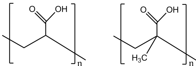
Slika 18. Strukturni prikaz ( lijevo ) poli(akrilne kiseline) i ( desno ) poli(metakrilne kiseline).
