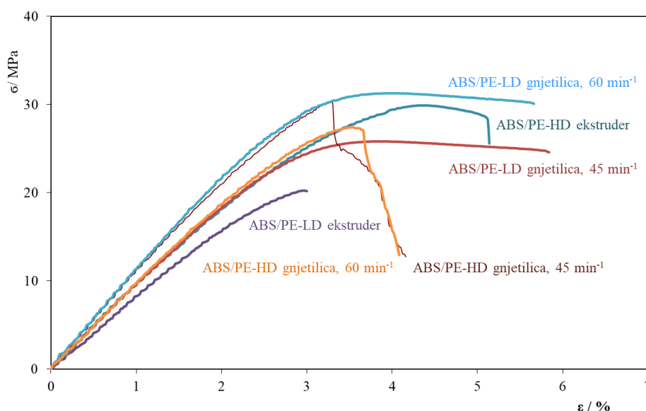
Slika 38. Grafički prikazi ovisnosti naprezanja o istezanju za polimerne mješavine s ABS-om omjera 90/10 pripremljene u ekstruderu i u gnjetilici
