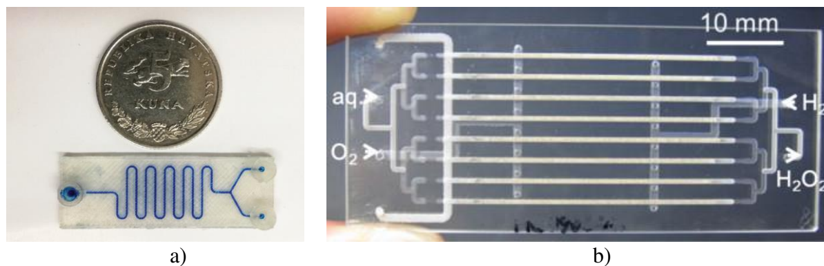
Slika 1. Mikoreaktori: a) mikroreaktor izrađen od čistoga polilaktida [1], b) stakleni mikroreaktor [21]
