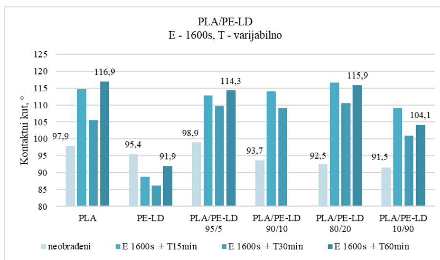
Slika 52. Izmjereni kontaktni kutovi kod polimernih mješavina PLA/PE-LD pripremljenih u ekstruderu pri različitim uvjetima obrade CF_x -om (E – jetkanje; T – prevlačenje CF_x -om)
