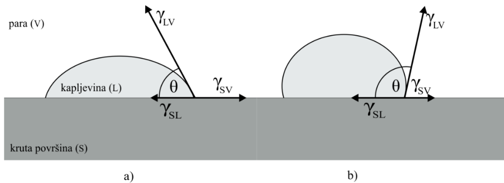
Slika 9. Kapljevina koje kvase (a) i koje ne kvase krutinu (b)
