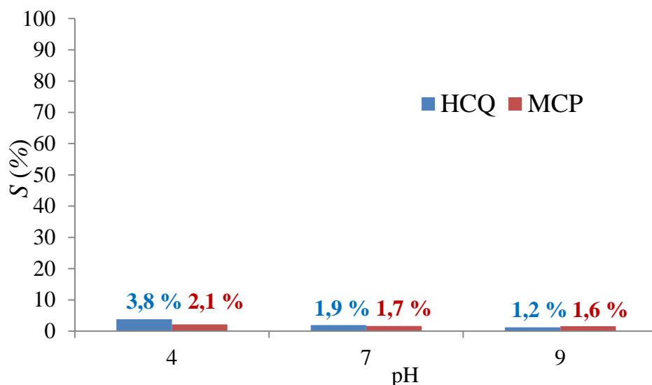
Slika 30. Hidrolitička stabilnost hidroksiklorokina ( c_0(\text{HCQ}) = 3,0 \cdot 10^{-5} \text{ mol L}^{-1} ) i metoklopramida ( c_0(\text{MCP}) = 3,3 \cdot 10^{-5} \text{ mol L}^{-1} ) pri 50 °C tijekom pet dana
