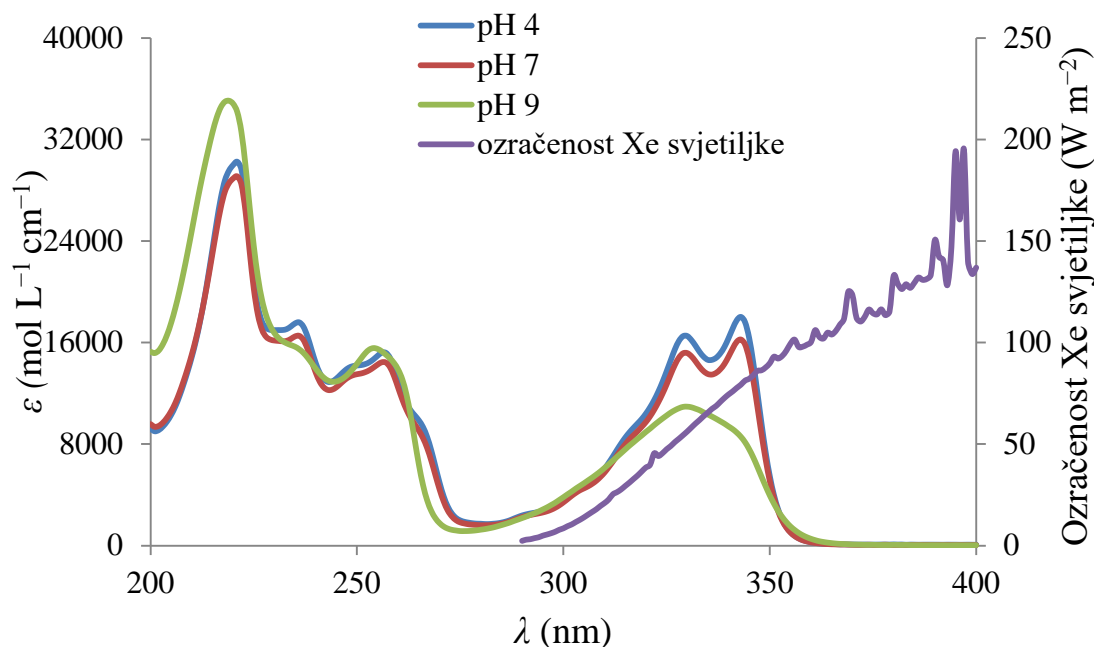
Slika 36. Apсорpcijski spektri hidroksiklorokina ( c_0 = 3 \cdot 10^{-5} \text{ mol L}^{-1} , b = 1 \text{ cm} ) pri pH 4, 7, 9 i spekter ozračenosti ksenonske svjetiljke
