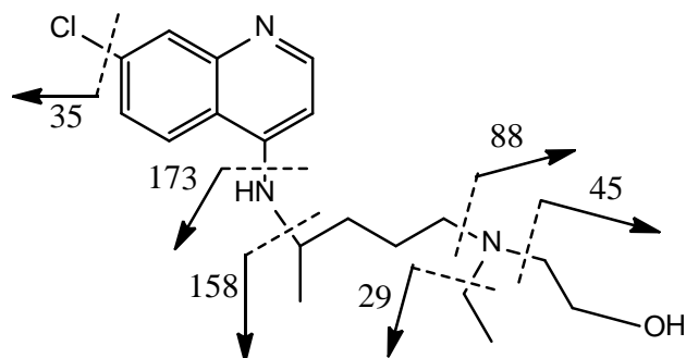
Slika 41. Predloženi fragmentacijski putevi razgradnje molekularnog iona hidroksiklorokina ( m/z = 336 )
