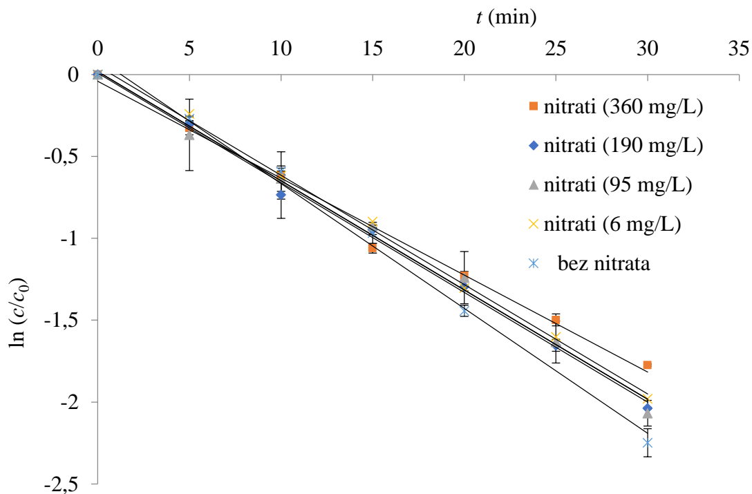
Slika 17.P Utjecaj nitrata na kinetiku fotolitičke razgradnje metoklopramida
