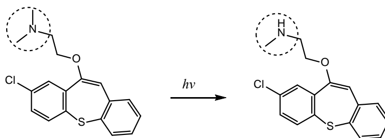
Slika 18. Primjer dealkilacije zotepina i nastanak njegovog fotoproizvoda (preuzeto iz [196])
