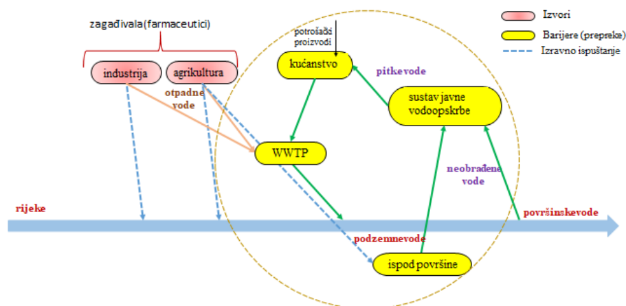
Slika 3. Shema toka zagađivača (farmaceutika) iz različitih izvora [40]
