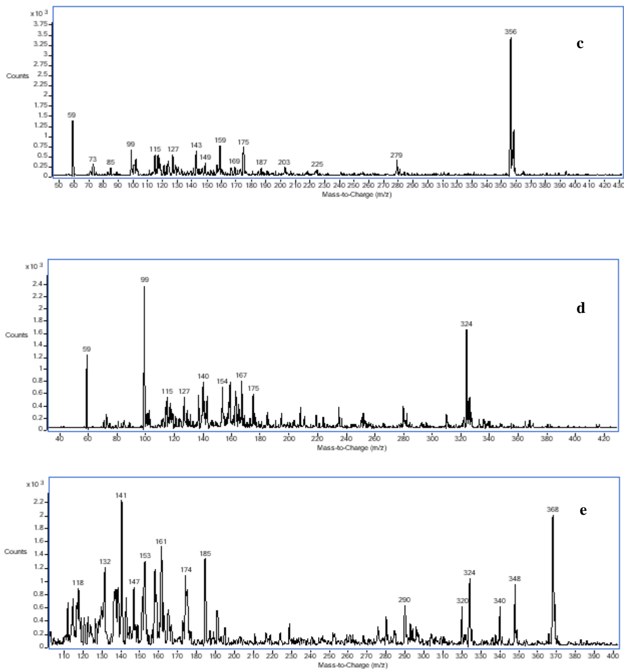
Slika 12. P Spektri masa za detektirane razgradne fotoproducte hidroksiklorokina u pozitivnom načinu rada ( a, b pH = 4, 18 h osvjetljavanja; c za 36 h osvjetljavanja ; d, e za pH = 9 nakon 10 min osvjetljavanja; Xe svjetiljka, 500 W m -2 )
