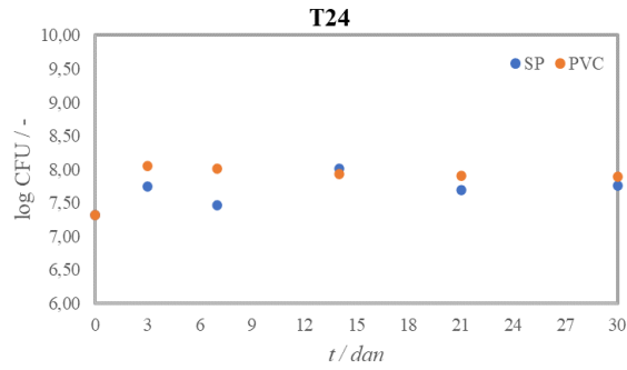
Slika 4.2. Promjena logaritamske vrijednosti CFU tijekom 30 dana trajanja biorazgradnje MP PVC-a primjenom Bacillus subtilis za pokuse s OG od 0,3: a)T1, b)T7, c)T13, d)T15, e)T16, f)T17, g)T18, h)T21 te i)T24.
