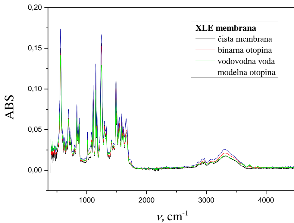
Prilog 10. FTIR spektar ispitivane XLE membrane za acetamidrid
