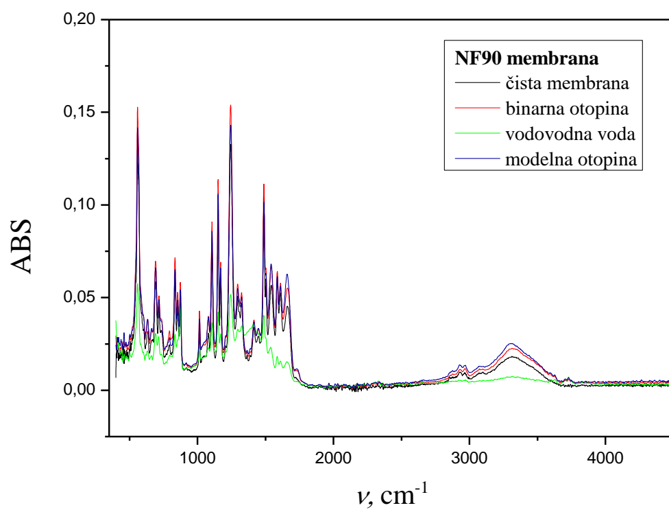
Prilog 9. FTIR spektar ispitivane NF90 membrane za acetamidrid
