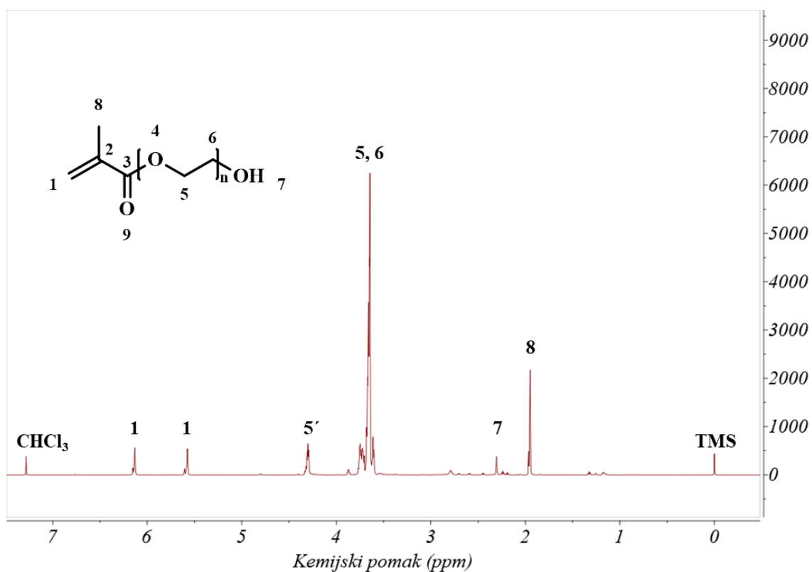
Slika 42. ^1\text{H} NMR spektar PEG-MA
