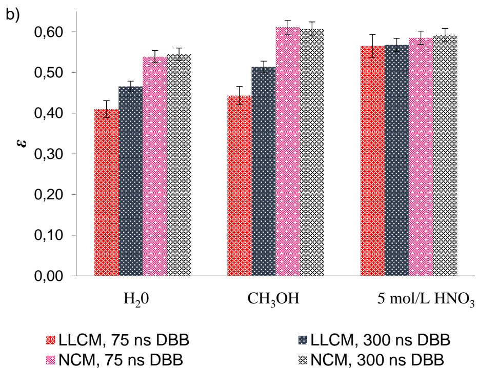
Slika 45. Učinkovitost detekcije Čerenkovljevim brojenjem a) ^{89}\text{Sr} b) ^{90}\text{Sr} - ^{90}\text{Y} u različitim otapalima. 16 mL uzorka u plastičnim bočicama. DBB je 75 ns i 300 ns u LLCM-u i NCM-u.
