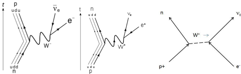
Slika 3. Feynmanovi dijagrami \beta^- , \beta^+ i EZ raspada [7].
