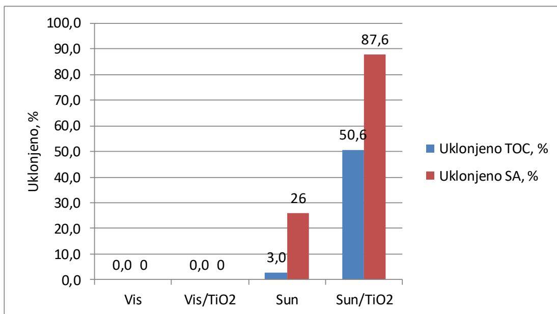
Slika 4.6. Prikaz uklanjanja SA i organskog ugljika u fotoreaktoru R2. Početni uvjeti procesa c_{sa} = 0,2 \text{ mmol dm}^{-3} , \text{pH } 3 , \gamma_{\text{TiO}_2\text{-P25}} = 1 \text{ g dm}^{-3} . Rezultati uzimaju u obzir smanjenje koncentracije SA i organske tvari nakon uspostavljanja ravnotežne adsorpcije.
