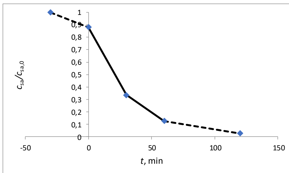
Slika 4.25. Prikaz fotokatalitičkog procesa \text{FeCl}_3 //UV-C/ \text{TiO}_2 . Početni uvjeti c_{sa} = 0,2 \text{ mmol dm}^{-3} , \text{pH } 3 , \gamma_{\text{TiO}_2\text{-P25}} = 1 \text{ g dm}^{-3} . Proces je proveden u fotoreaktoru R1 pri UV-C zračenju. Proces se odnosi na prikaz preostale koncentracije SA u suspenziji ili otopini izmjerenoj u R1 fotoreaktoru. Od -30 do 0 min prikazana je adsorpcija SA na površinu fotokatalizatora (proces u mraku), u 0 min dodan je koagulant c_{\text{FeCl}_3 \times 6 \text{ H}_2\text{O}} = 1,88 \text{ mmol dm}^{-3} , od 0 do 60 min proveden je fotokatalitički proces, a od 60 do 120 min podešen je pH na 7 radi pokretanja procesa taloženja.
