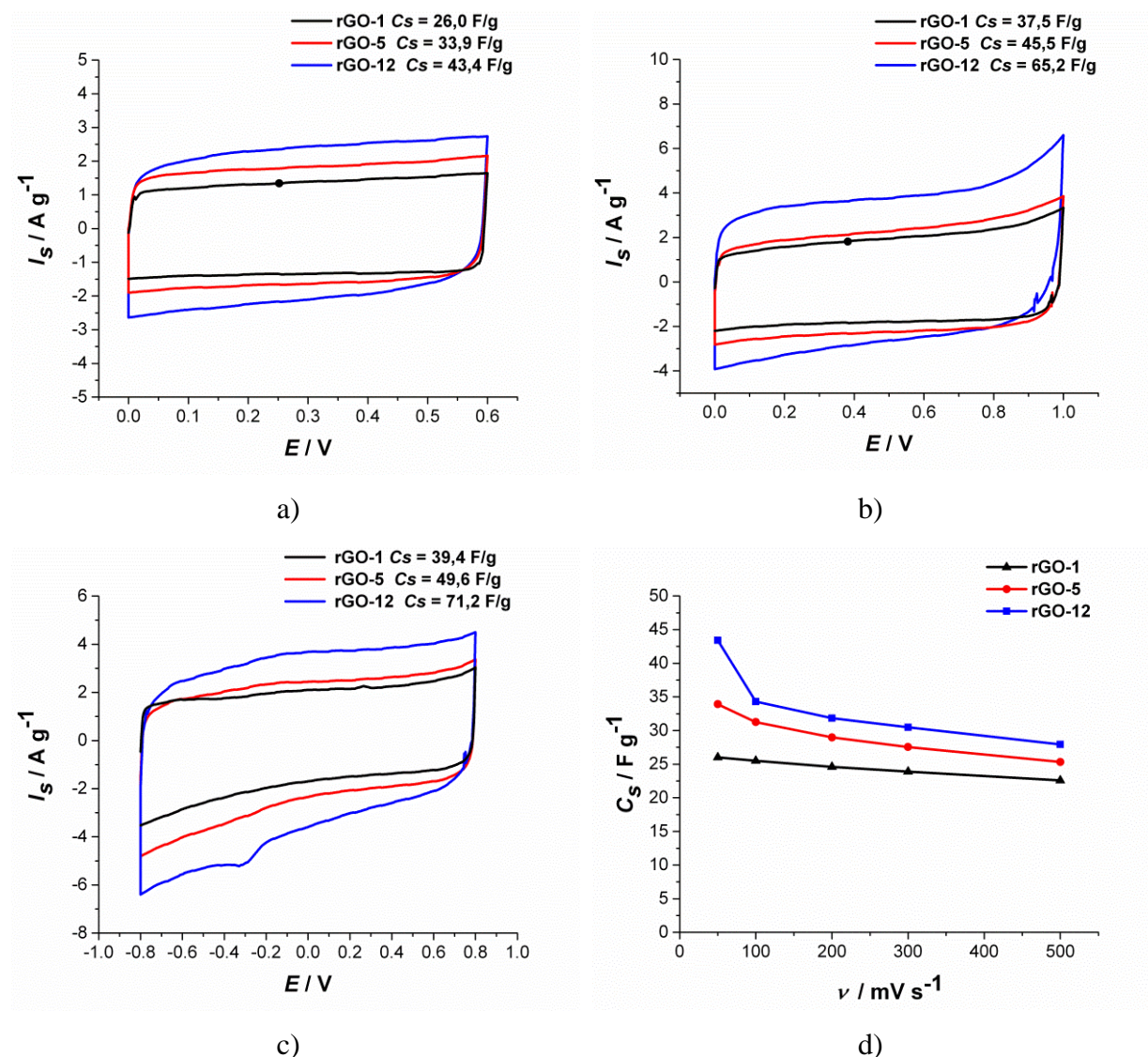
Slika 5.2. Ciklički voltamogrami zabilježeni za uzorak rGO-1, rGO-5 i rGO-12 u 0,5 mol dm -3 Na 2 SO 4 ; a, b i c) unutar različitih granica potencijala uz v = 50 mV s -1 i d) ovisnost specifičnog kapaciteta o brzini promjene potencijala za ispitivanje provedeno od 0 – 0,6 V.
