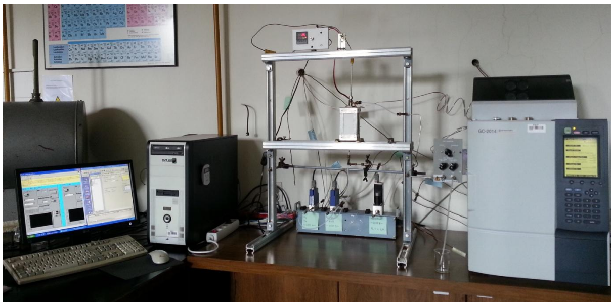
Slika 4.11 Eksperimentalna aparatura
