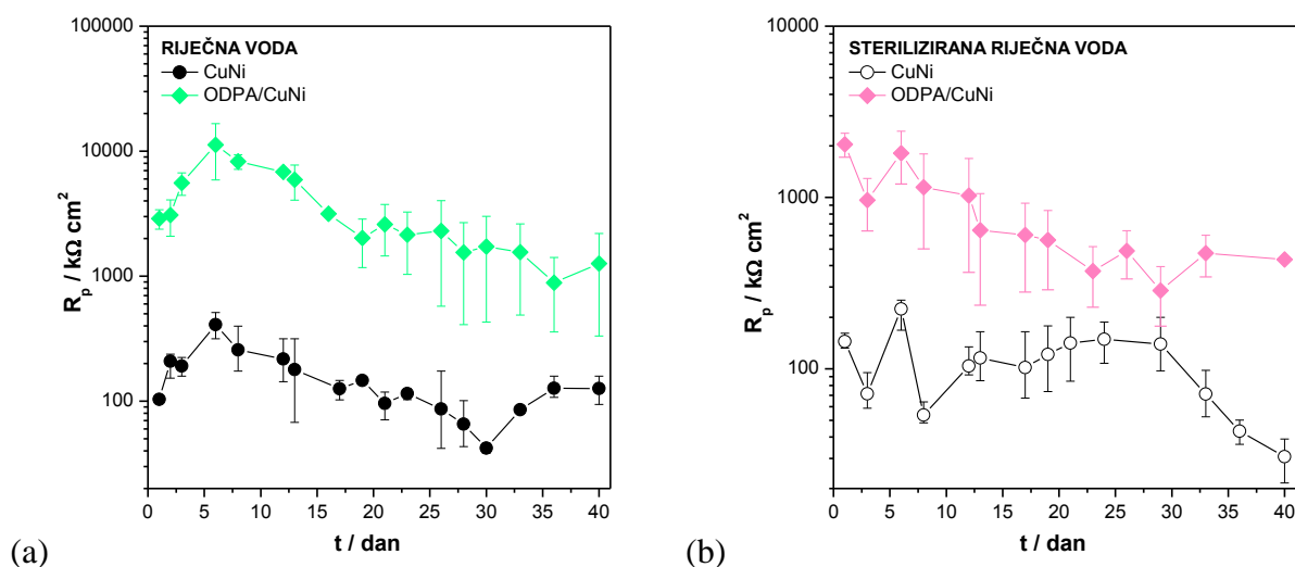
Slika 4.83. Ovisnost polarizacijskog otpora o vremenu za netretirane i tretirane uzorke u: (a) prirodnoj te (b) steriliziranoj riječnoj vodi.
