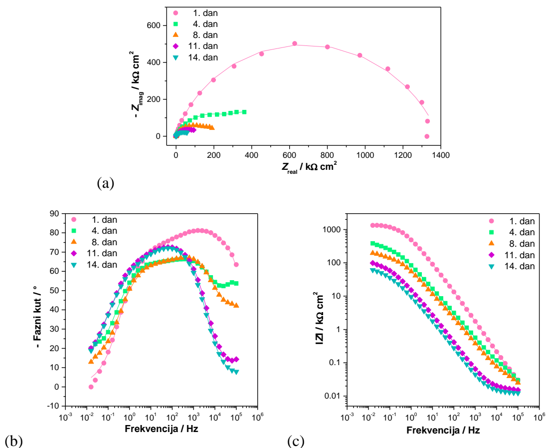
Slika 4.20. Impedancijske krivulje za H-T40 uzorak: (a) Nyquistov prikaz, (b) i (c) Bodeov prikaz (simboli – eksperimentalni podaci, linije – rezultati dobiveni iz modela).
