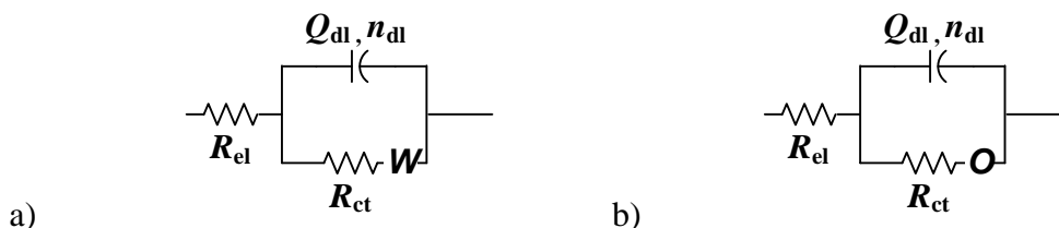
Slika 4.101. Ekvivalentni električni krugovi korišteni za usklađivanje EIS spektara netretiranog CuNi uzorka.
