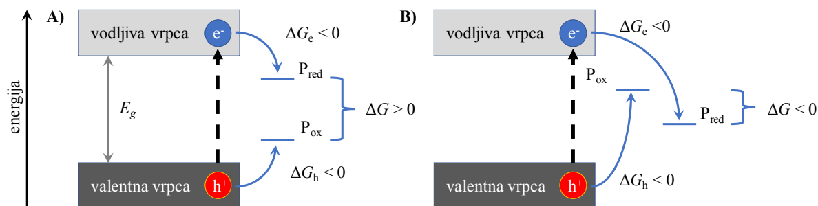
Slika 2.9. Elektronska struktura fotokatalizatora uz primjer A) termodinamički nespontane reakcije ( \Delta G > 0 ) te B) spontane reakcije ( \Delta G < 0 ) tijekom fotokatalize.
