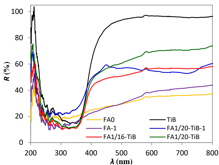
Slika 4.8. UV/Vis spektri čistih komponenti, sintetiziranog \text{TiO}_2 i uzorka lebdećeg pepela (FA1) te FA1/ \text{TiO}_2 nanokompozitnih fotokatalizatora.
