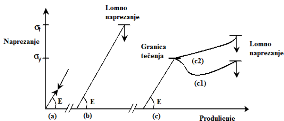
Slika 4. Makroskopski prikaz napreznja: (a) reverzibilna plastična deformacija (b) pucanje lomljivog materijala, (c) rastezljivo ponašanje 15
