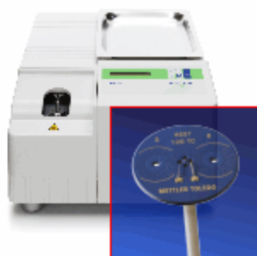
Slika 3.4. Diferencijalni pretražni kalorimetar
