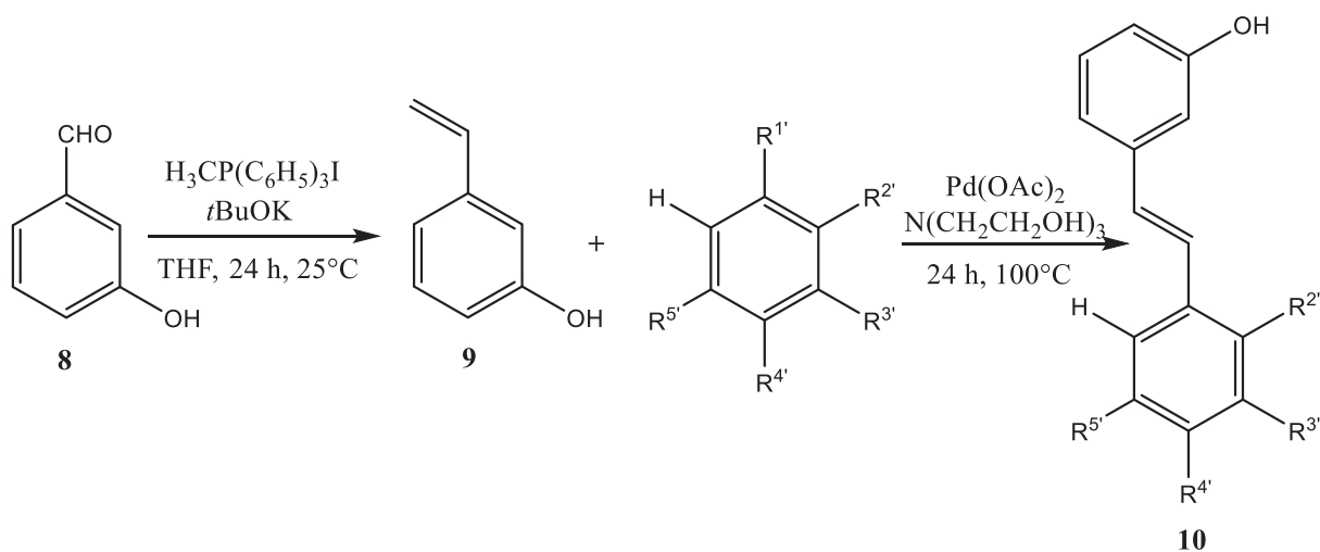
Shema 5. Sinteza supstituiranog stirena Wittigovom olefinacijom i 3-hidroksisupstituiranog stilbena uzastopnom Mizoroki-Heckovom reakcijom
