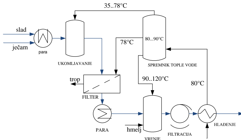
Slika 11. Procesna shema toplog dijela proizvodnje piva
