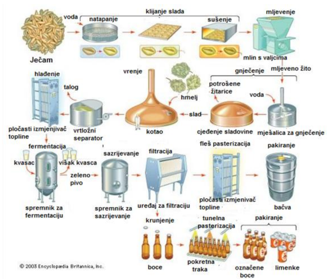
Slika 8. Proces proizvodnje piva
