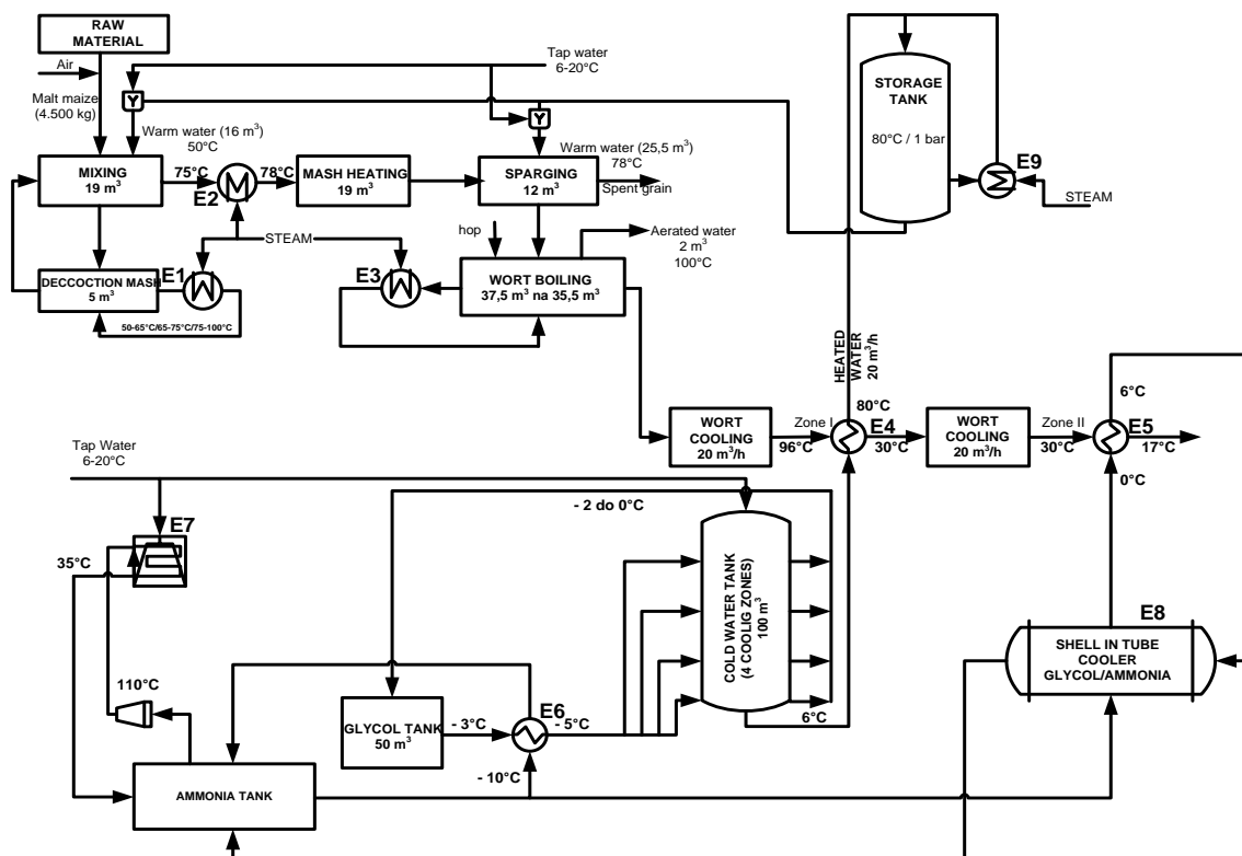
Slika 13. Procesna shema proizvodnje piva
