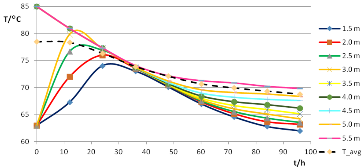
Slika 20. Promjena temperature segmenata spremnika s vremenom - proljeće
