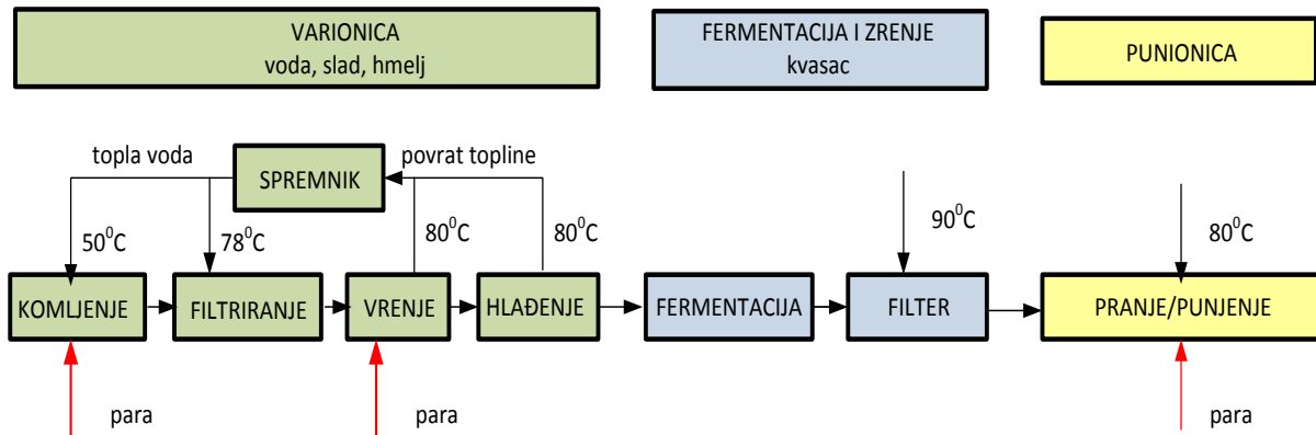
Slika 9. Glavni dijelovi proizvodnog procesa
