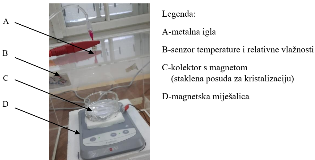
Slika 5.2. Prikaz dijela aparature u komori za pripremu mikrosfera metodom elektroštrcanja.
