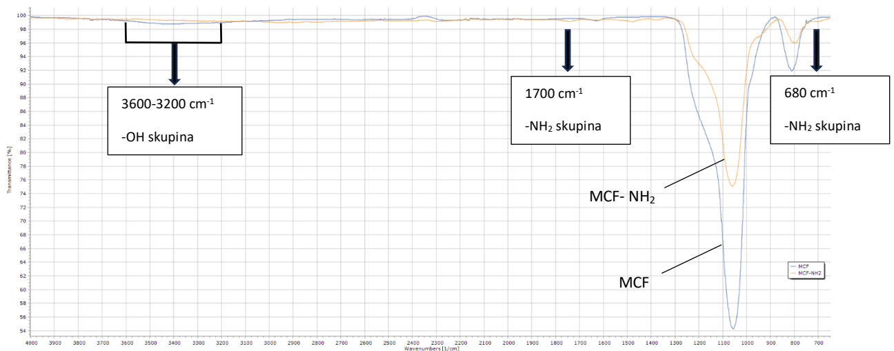
Slika 30. FTIR spektrogram funkcionalizirane i aktivirane te nefunkcionalizirane mezoporozne silike
