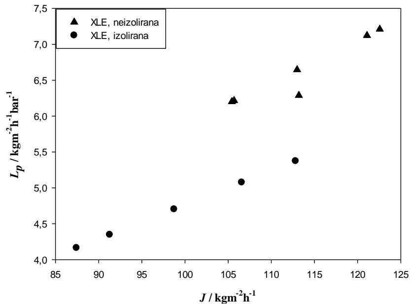
Slika 21. Usporedba neizolirane i izolirane XLE membrane
