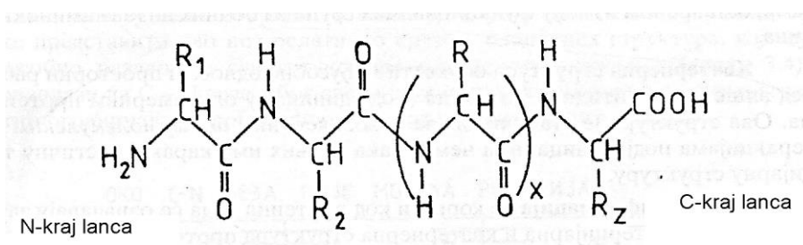
Slika 2. Peptidni lanac [13]
