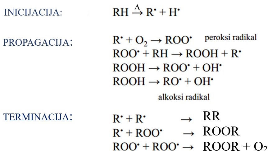
Slika 2.6. Mehanizam toplinske razgradnje polimera
