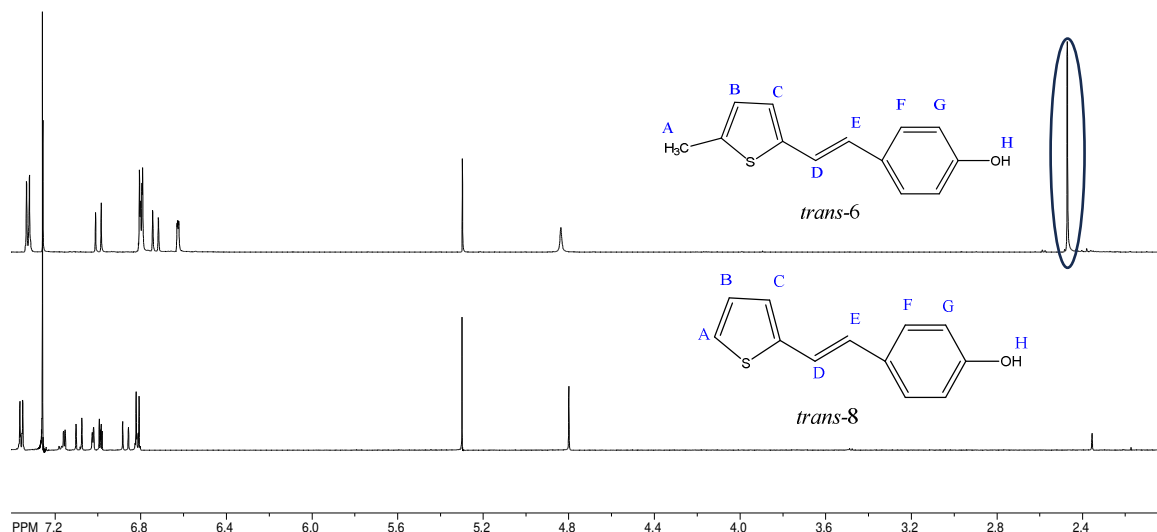
Slika 12. 1 H NMR spektri i strukture trans-6 i trans-8 izomera.
