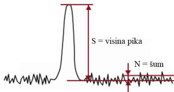
Slika 7. Grafički prikaz SNR parametra [7]
