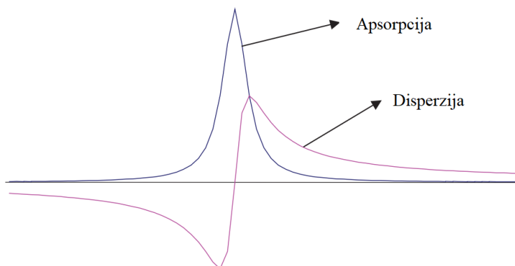
Slika 31. Oblici linija apsorpcije i disperzije
