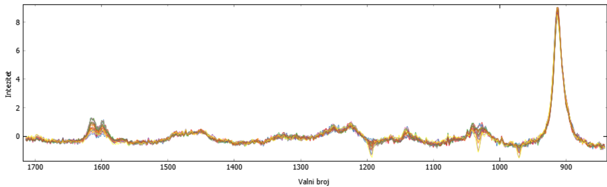
Slika 53. Uklanjanje bazne linije temeljene na asimetričnoj metodi najmanjih kvadrata na neobrađenom spektru i skaliranje SNV metodom
