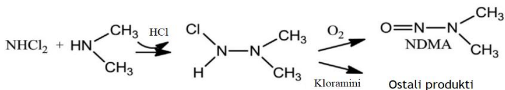
Slika 4. Nukleofilna supstitucija između dikloramina i sekundarnog amina te nastanak N -nitrozamina (NDMA) [14]
