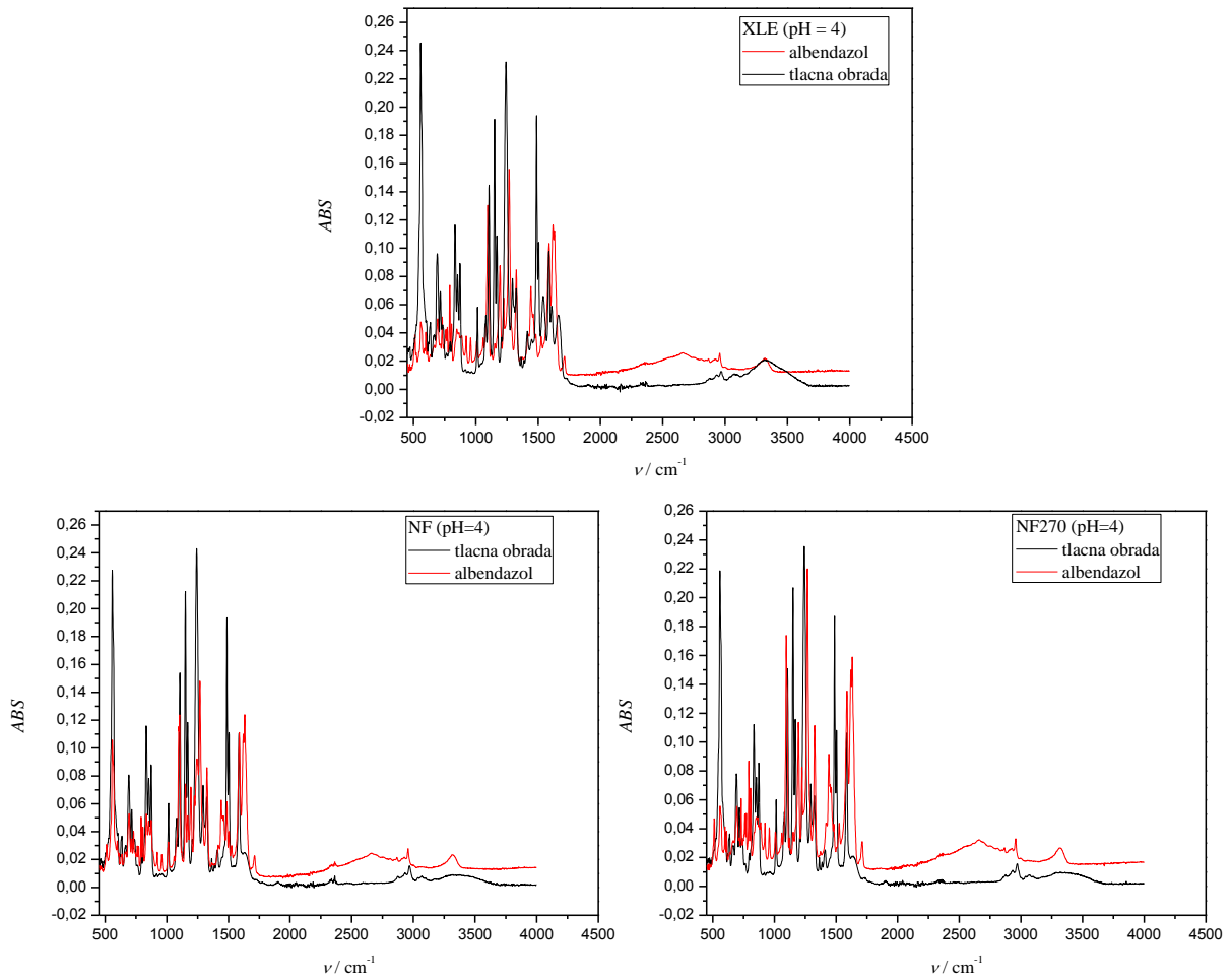
Slika 4.10. FTIR spektar za XLE, NF, i NF270 membrane nakon tlačne obrade i tretmana otopinom alabendazola.
