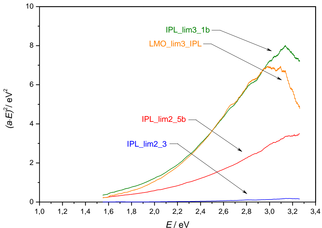
Slika 16. Taucov graf (ovisnost umnožka (\alpha \cdot E)^2 o energiji fotona, E ) za tanke filmove \text{LaMnO}_3
