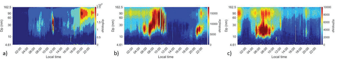
Prilog 2. Prikaz preostalih konturnih dijagrama za dane s događajima povezanim s onečišćenjem po datumima a) 20. ožujka 2023. b) 7. travnja 2023. c) 8. travnja 2023.
