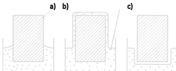
Slika 3. Prikaz a)vlaženja, b)razlijevanja i c)odvajanja
