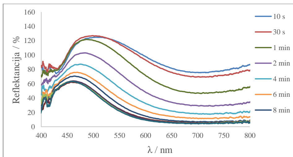
Slika 23. Reflektancijski spektar dobiven ispitivanjem utjecaja vremena izlaganja papirnih traka UV zračenju na razvoj nanočestica berlinskog modrila na papiru.
