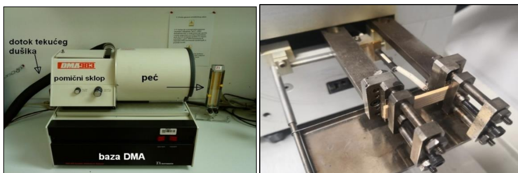
Slika 25. DMA analizator , DMA 983 TA Instruments,USA
