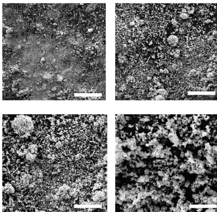
Slika 20. CdS/SBA-15 (20% CdS)
