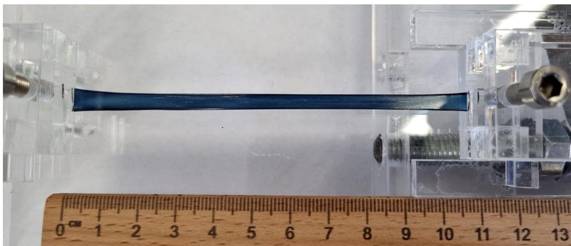
Slika 48. Maksimalno istezanje filma PEDOT-Br:S-SEBS
