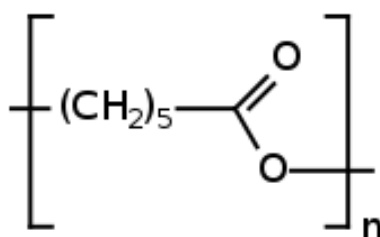
Slika 2.10. Struktura PCL-a [34]
