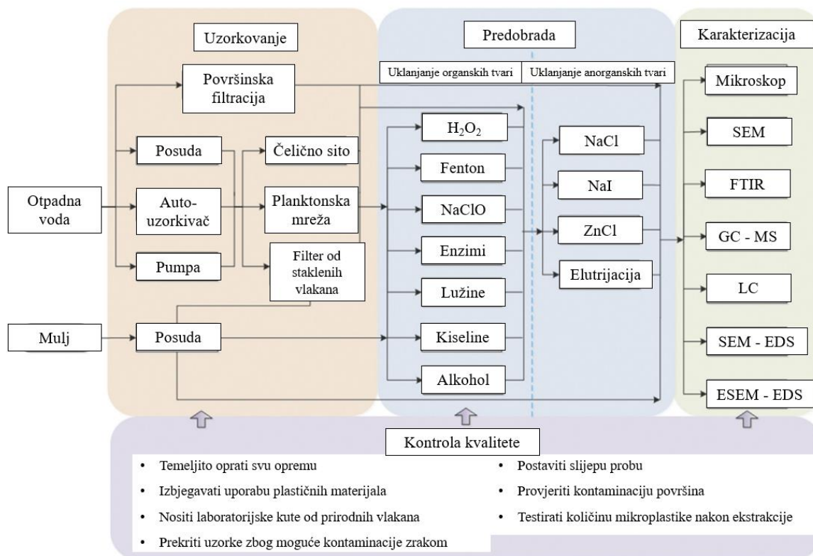
Slika 6. Dijagram toka koji prikazuje sažetak koraka i tehnika korištenih za detekciju mikroplastike u postrojenjima za obradu otpadnih voda [5]
