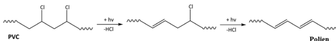
Slika 5. Dekloriranje PVC-a [7]
