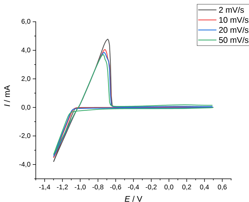
Slika 4.4. Ciklički voltamogrami zabilježeni tijekom depozicije cinka na rGO/20%CNT elektrodi pri različitim brzinama promjene potencijala u 2 mol dm -3 ZnSO 4
