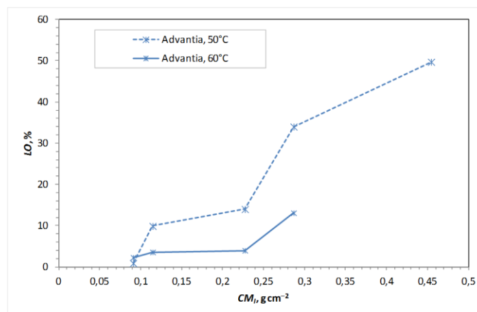
Slika 23. Dijagram promjene udjela loše obloženih tableta u preliminarnim eksperimentima [27]
